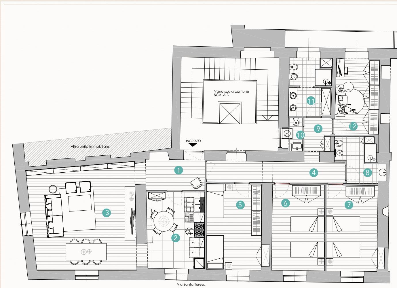
Planimetria generale
